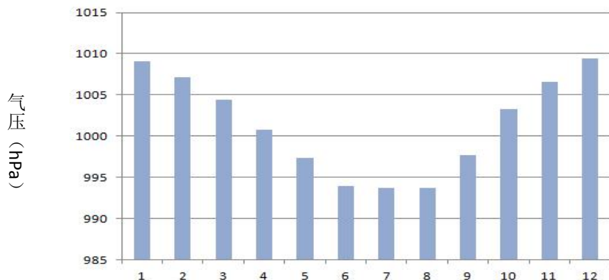
图 4-1 云浮国家气象站累年各月平均气压直方图
